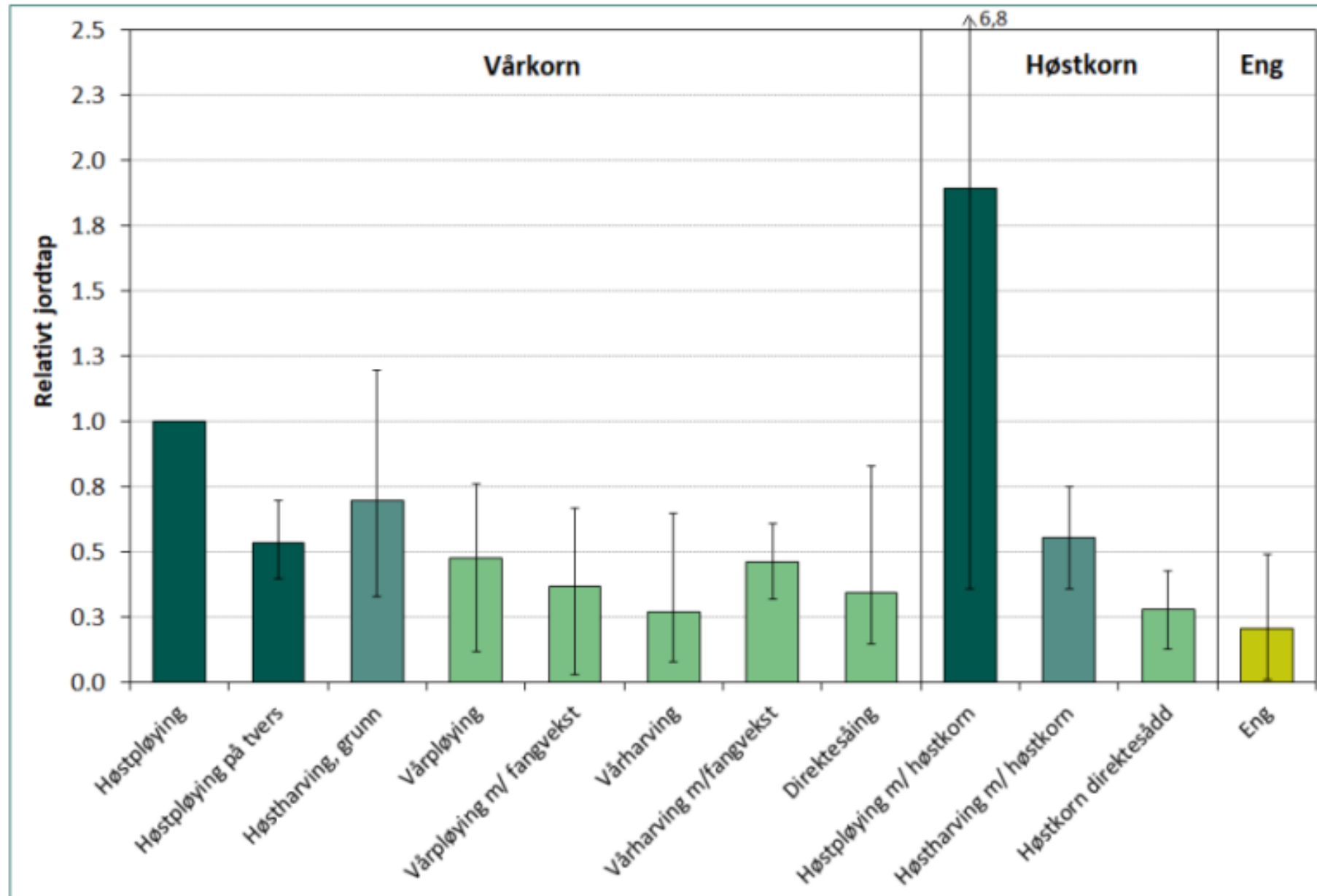
Figur 2: Gjennomsnittlig relativt jordtap ved ulike jordarbeidingsmetoder (Kværnø, Sigrun H. m.fl. 2020b, s. 4)
